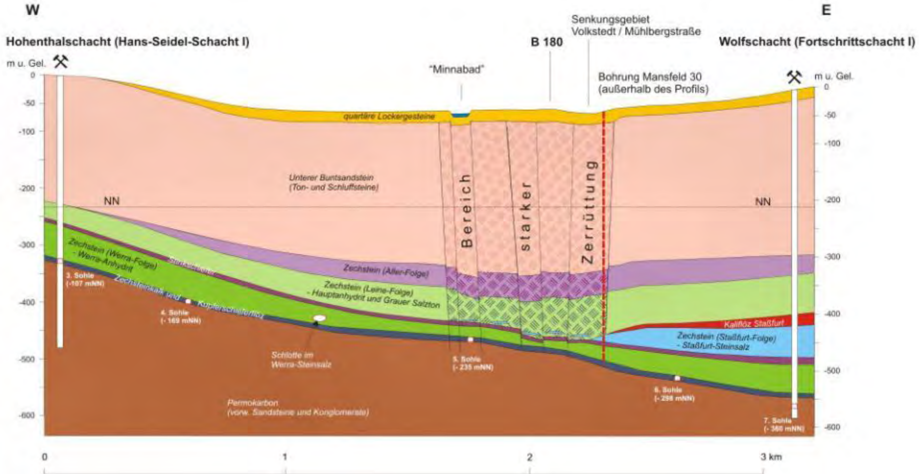
Geologischer Schnitt durch den Untergrund von Volkstedt
